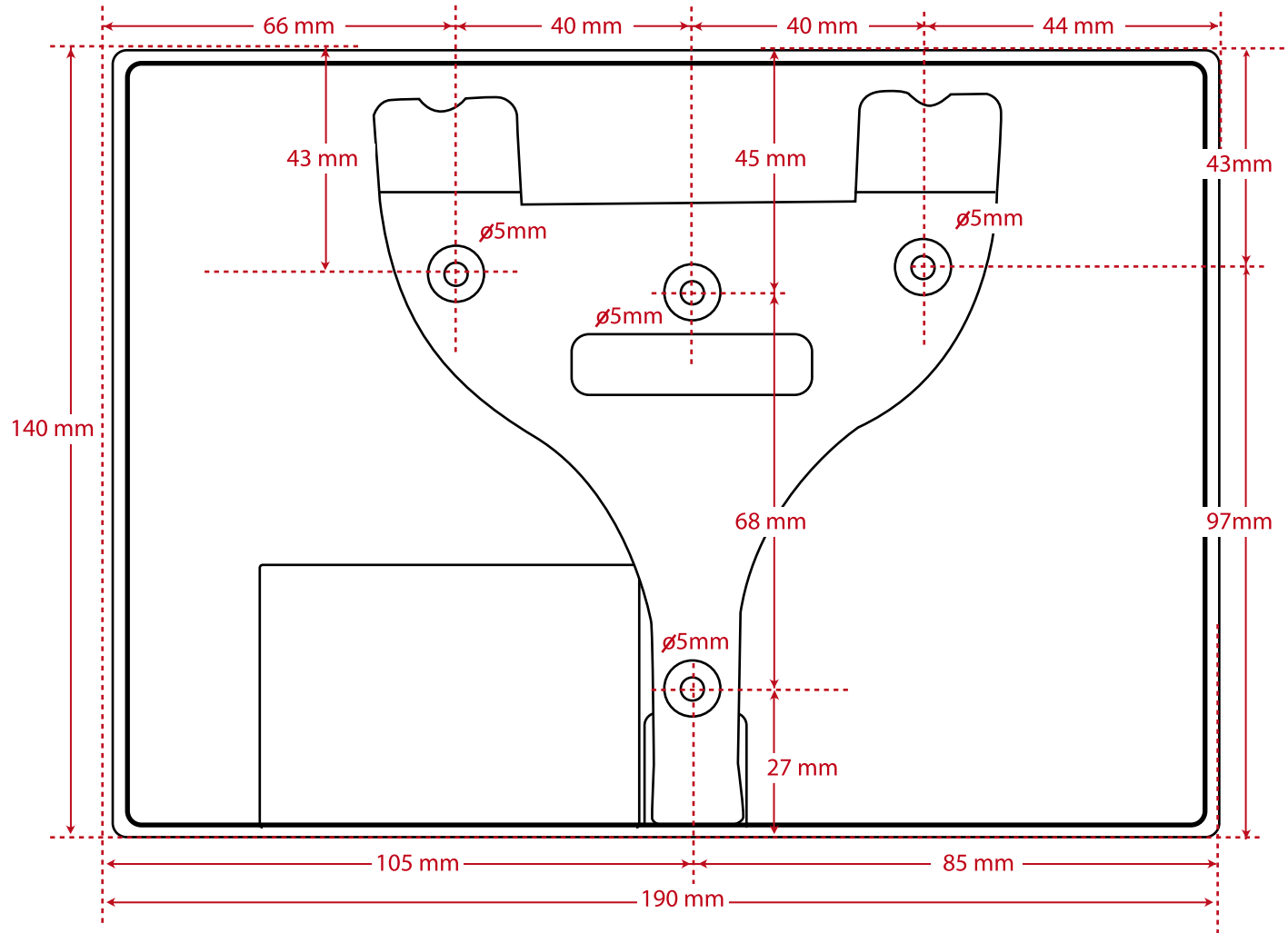
Vorderansicht des rückplatte
